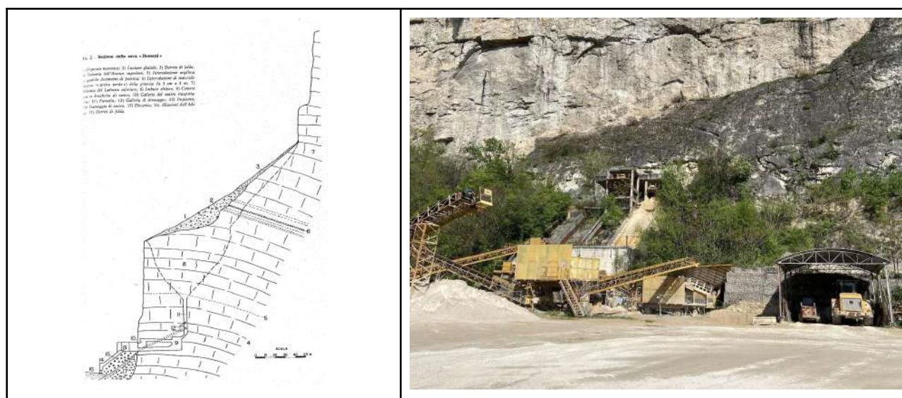
Fig. 4. A sinistra, una sezione geologica del versante su cui è impostata la miniera “Dosseni”, con riportata la sagoma dell’imbuto roccioso col fornello sul fondo e il raccordo con la galleria che si sviluppa pressoché orizzontale fino allo sbocco dalla parete rocciosa (1976). A destra, una vista, dal piazzale di lavorazione, della struttura in cemento armato presente allo sbocco della galleria (2023).
